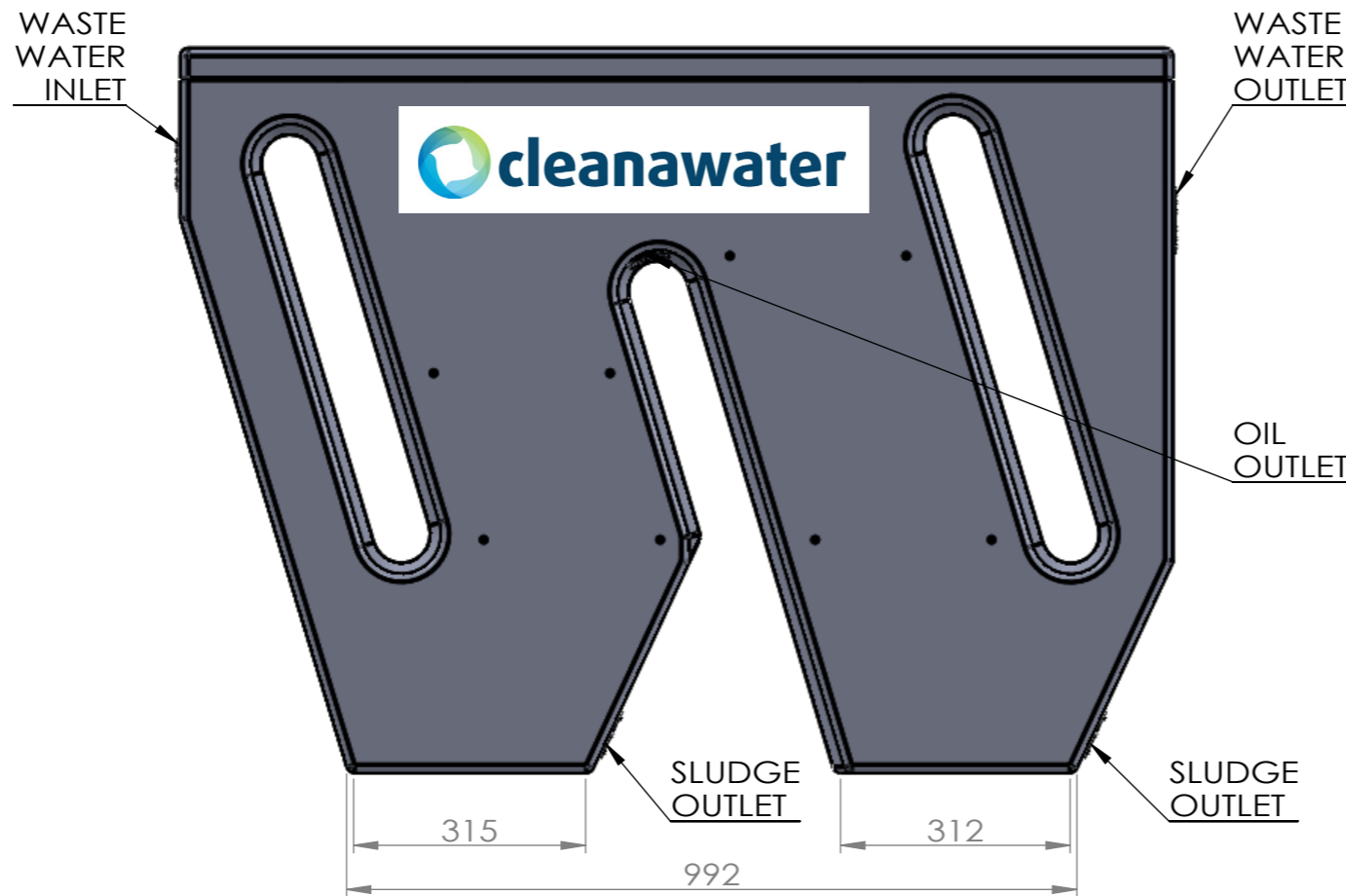
RIGHT ELEVATION
